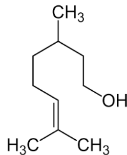
Gambar 1.1.2 Struktur sitranelol
