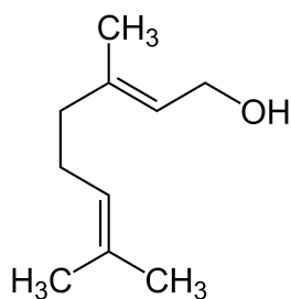
Gambar 1.1.3 Struktur Geraniol
